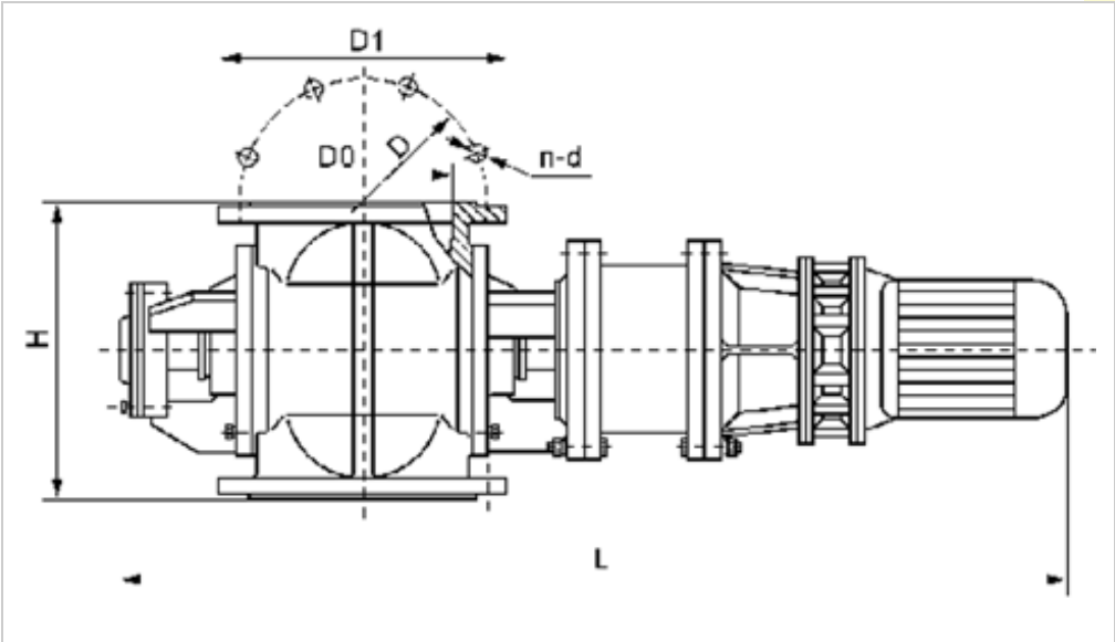
外型安装尺寸：
