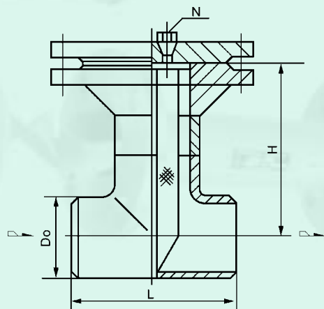
DGT I-W型
