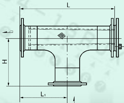
DGT III-F型
