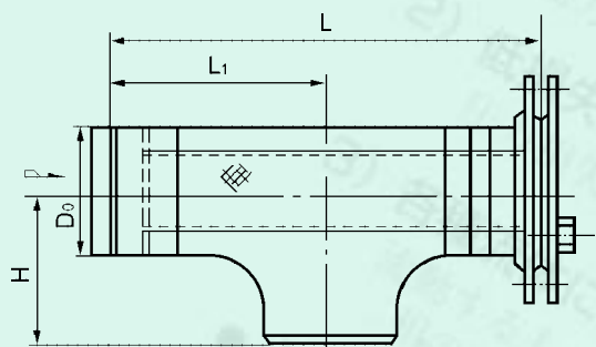
DGT II-W型
