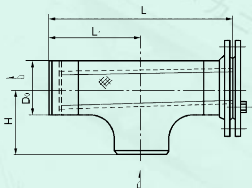
DGT III-W型
