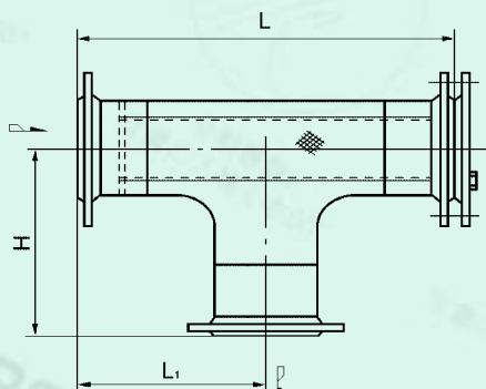
DGT II-F型
