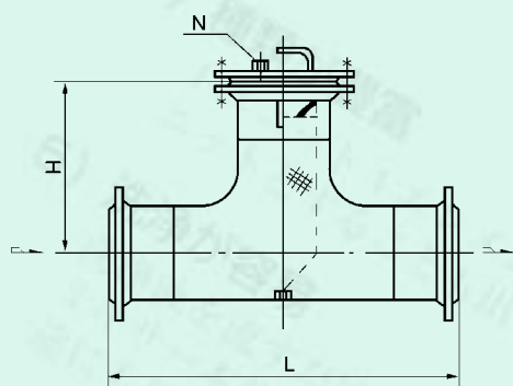
DGT I-F型
